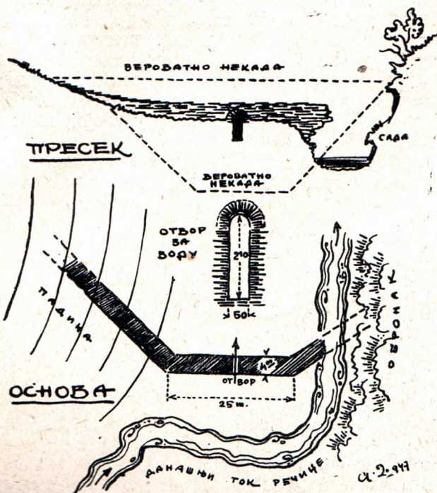
Сл. 12 Византиска водена брана код Царичина града. Le barrage sur la rivière à Caričin Grad.
